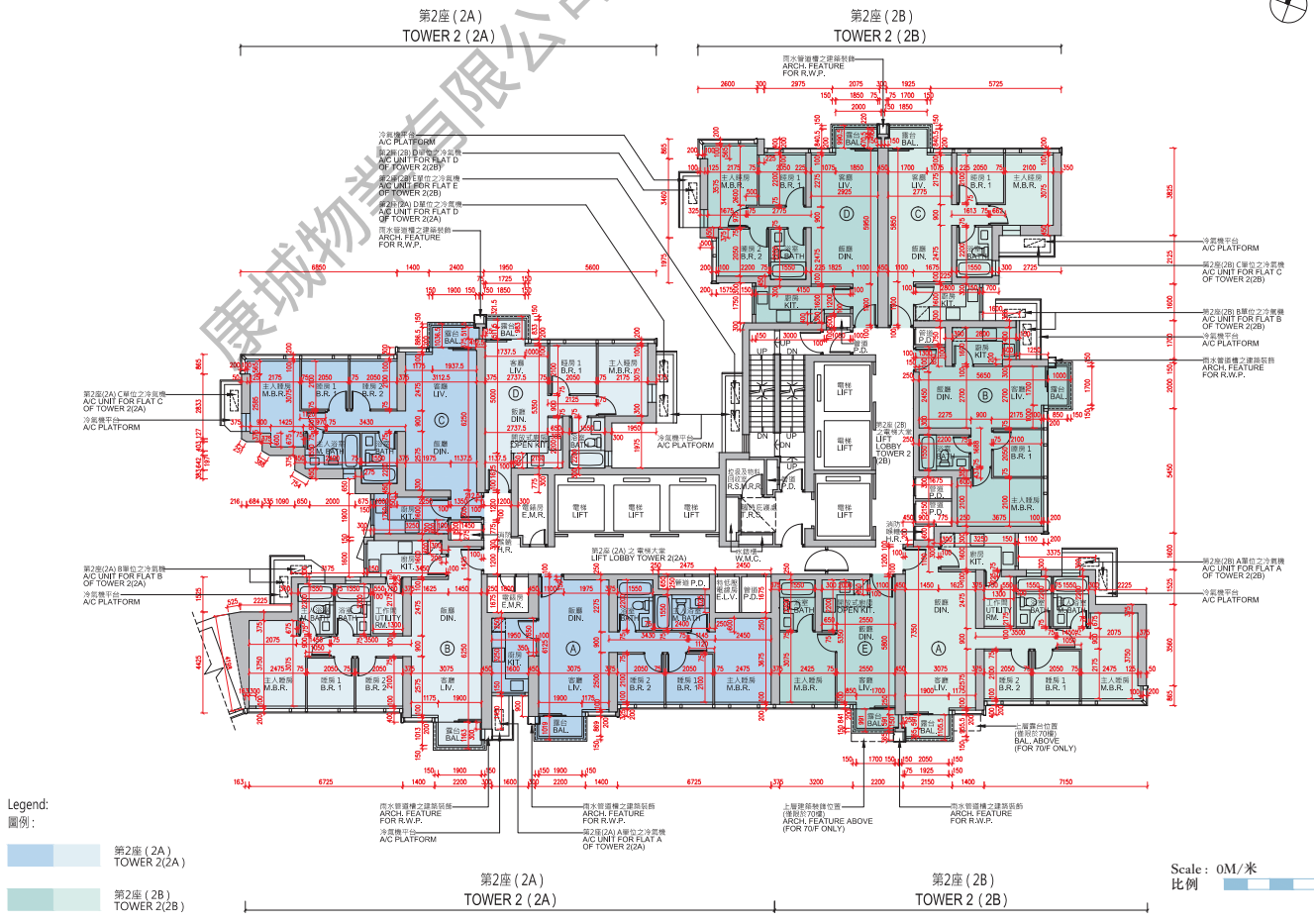
Tower 2(2A) & Tower 2(2B) 第2座(2A)及第2座(2B) 56/F-63/F, 65/F-69/F 56樓至63樓、65樓至69樓 Floor Plan 樓面平面圖
